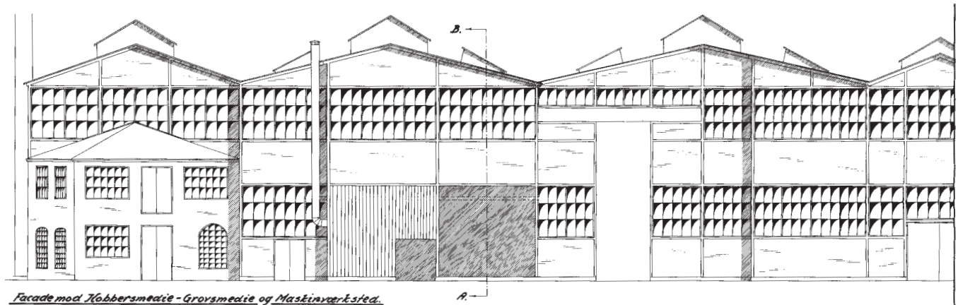
Facade mod Hobberrmedie - Grovsmedie og Maskinværksted.
